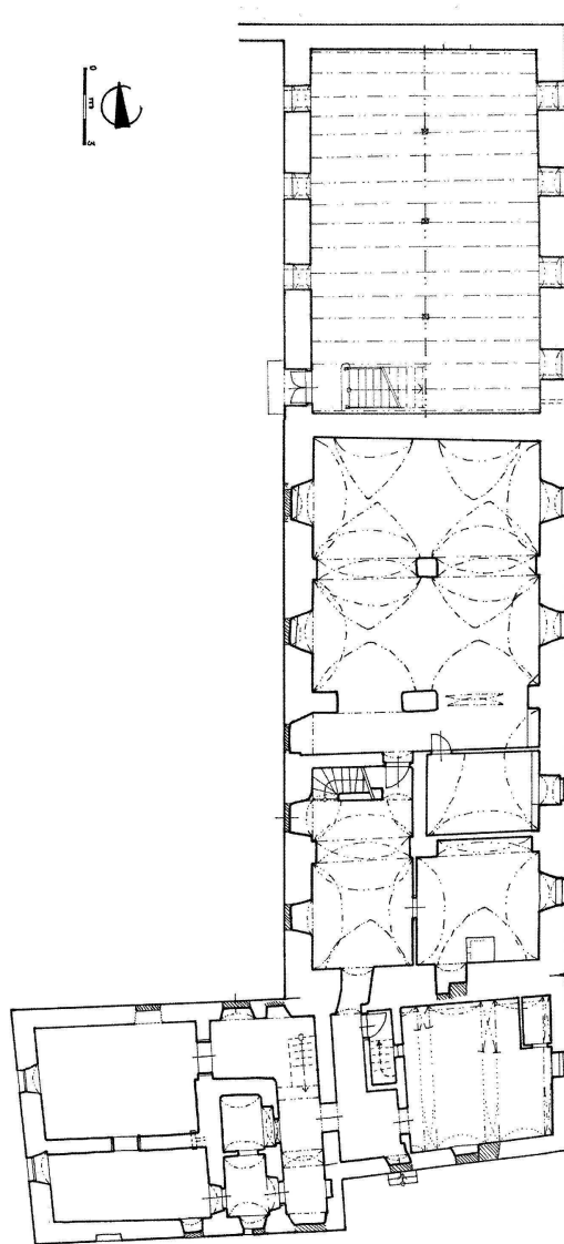
Obr. 3: Velká Polom (okr. Ostrava), půdorys přízemí sýpky čp. 164 (zaměření a kresba A. Knápek 2008).
