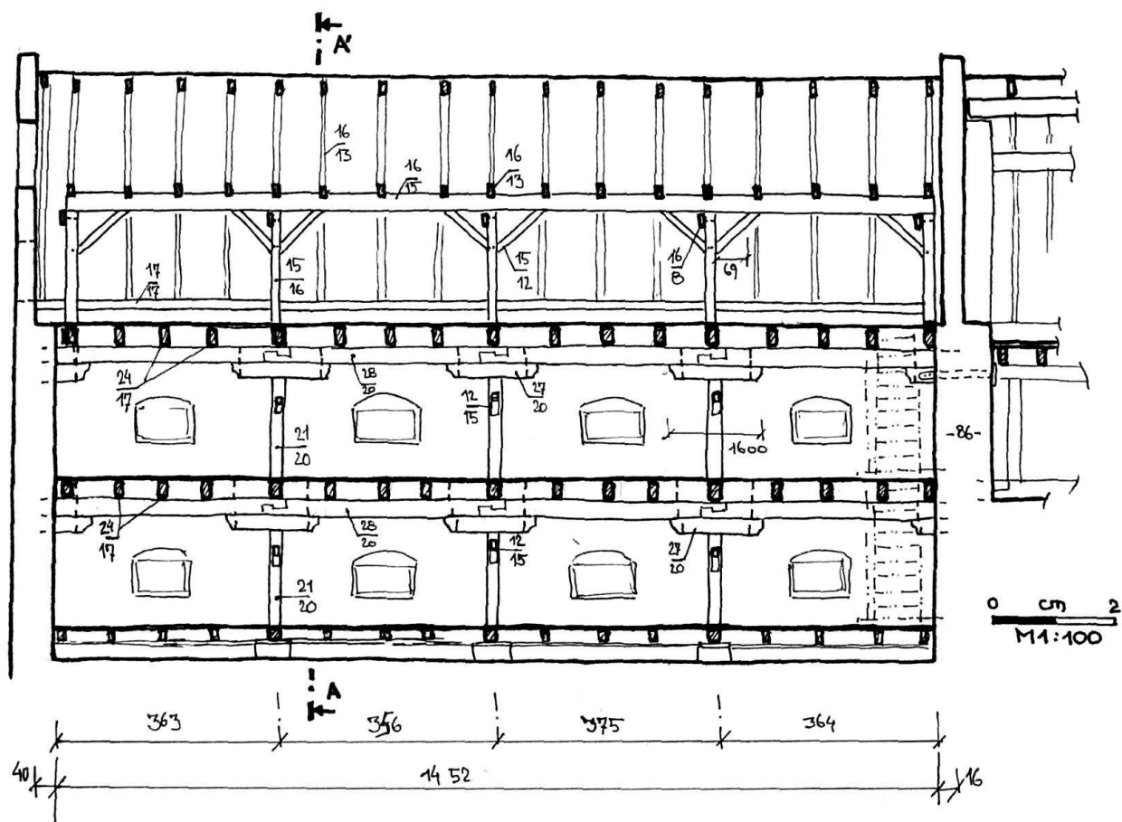
Obr. 4: Velká Polom (okr. Ostrava), podélný řez severní částí sýpky čp. 164 (zaměření a kresba A. Knápek 2008).
