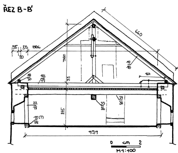
Obr. 6: Velká Polom (okr. Ostrava), příčný řez střední částí objektu čp. 164 (zaměření a kresba A. Knápek 2008).
