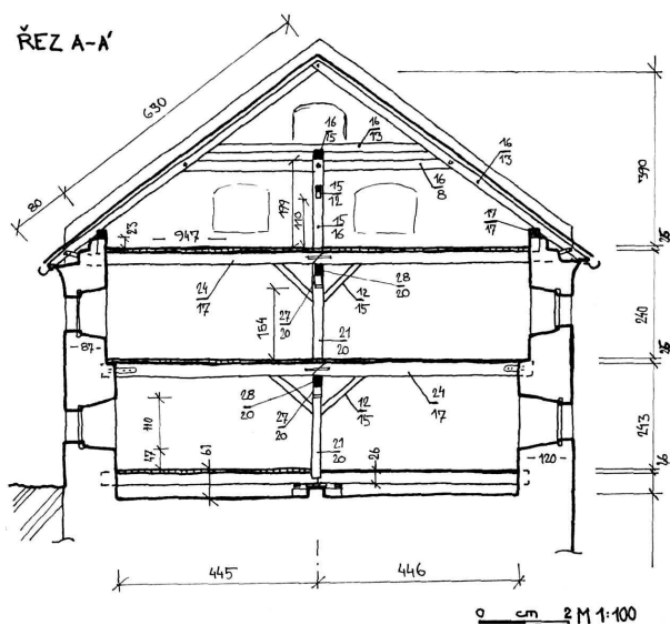
Obr. 5: Velká Polom (okr. Ostrava), příčný řez severní částí sýpky čp. 164 (zaměření a kresba A. Knápek 2008).
